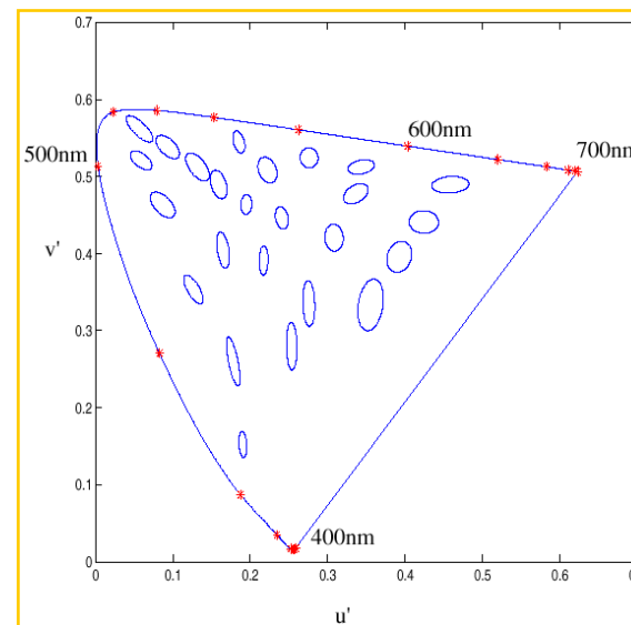
CIE u'v'
