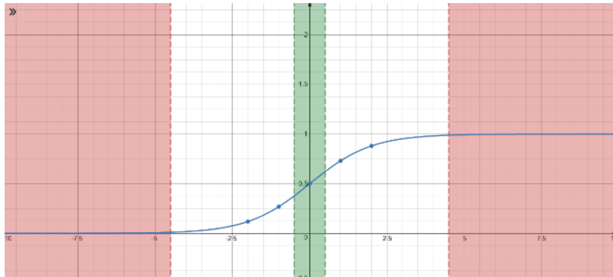
Sigmoid
