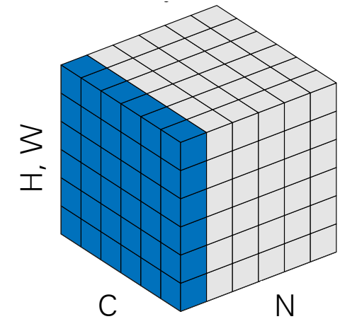
Layer Norm
